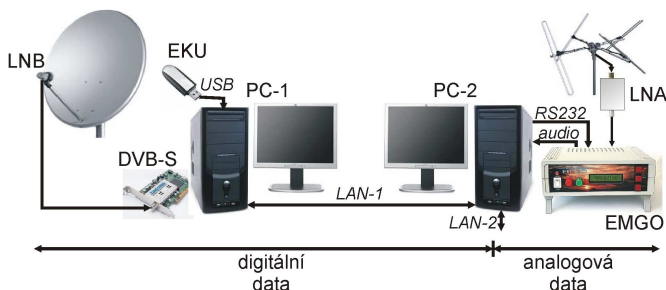
Obr. 4: Blokové znázornění přijímacího pracoviště
