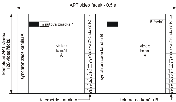
Obr. 1: Formát jednoho APT rámce [7]
