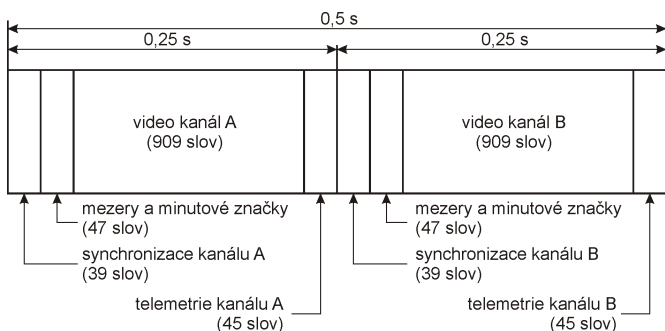
Obr. 2: Formát jednoho APT video řádku [7]
