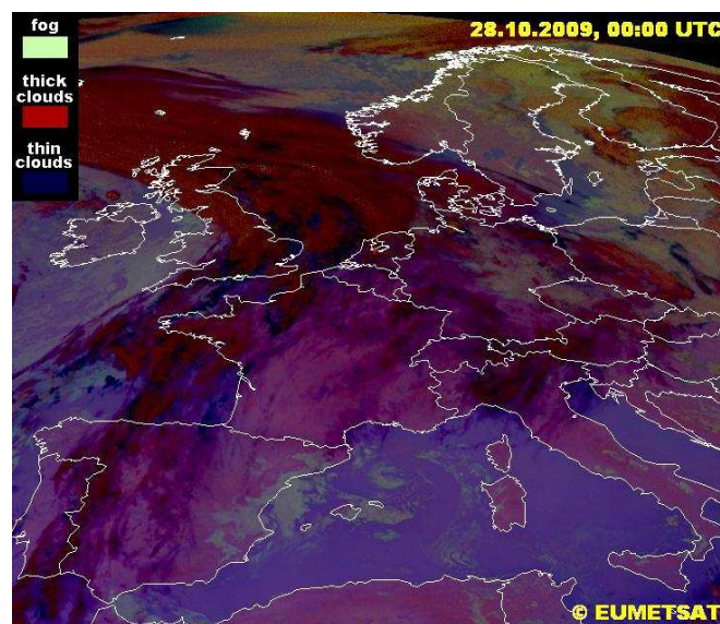
Obr. 6: Barevná kompozice tří kanálů radiometru SEVIRI (IR 3,9; IR 10,8, IR 12,0) pro noční detekci mlh, snímek ze dne 28. 10. 2009 ve 00:00 UTC. © EUMETSAT.
